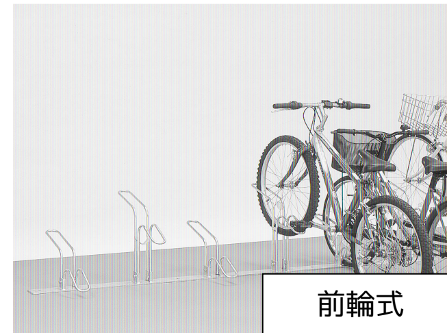
■前輪式 駐輪台数とレール長さ例
