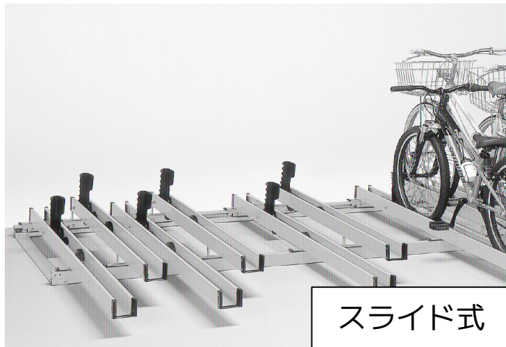
■スライド式 駐輪台数とレール長さ例
