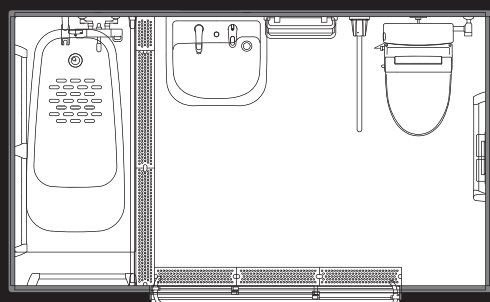
ユニバーサルツイン 浴室 平面図
